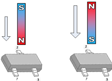
VOUT=低电平
