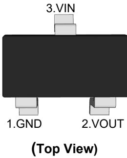
SOT-23-3
