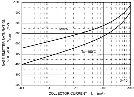
V_{BE} - I_c
