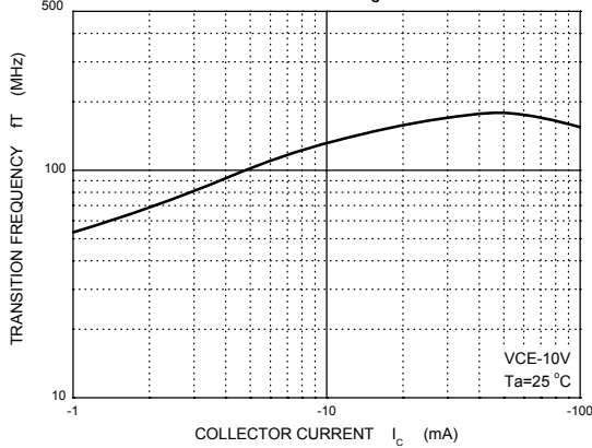
f_T - I_c
