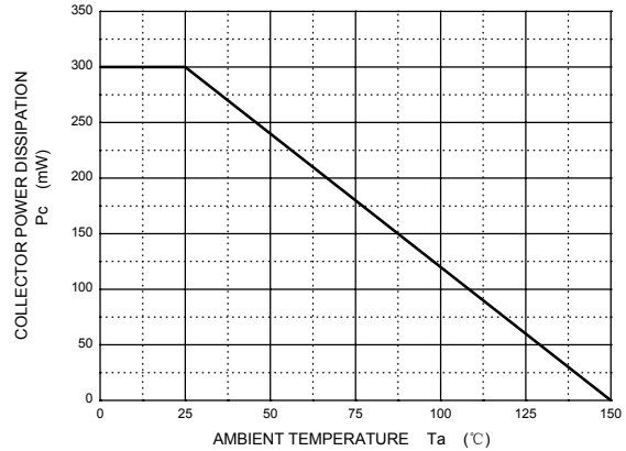
P_c - T_a
