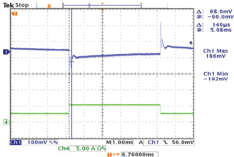
5%~50% Load Transient (AC) at 25°C@115V
