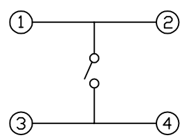
原理图
