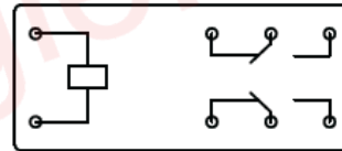
2转换 2C 型
