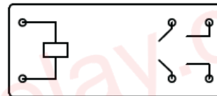
2常开 2A 型
