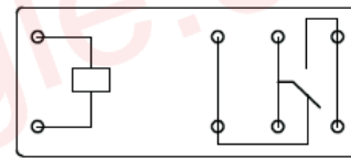
转换 C 型
