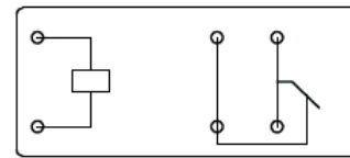
常闭B 型
