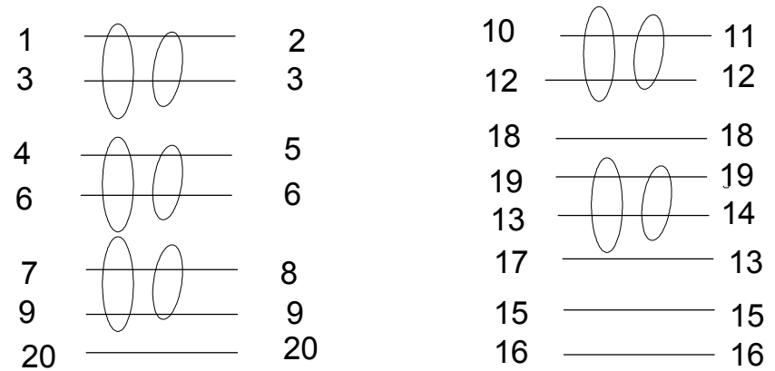
HDMI 19M MINI HDMI 19M HDMI 19M MINI HDMI 19M
