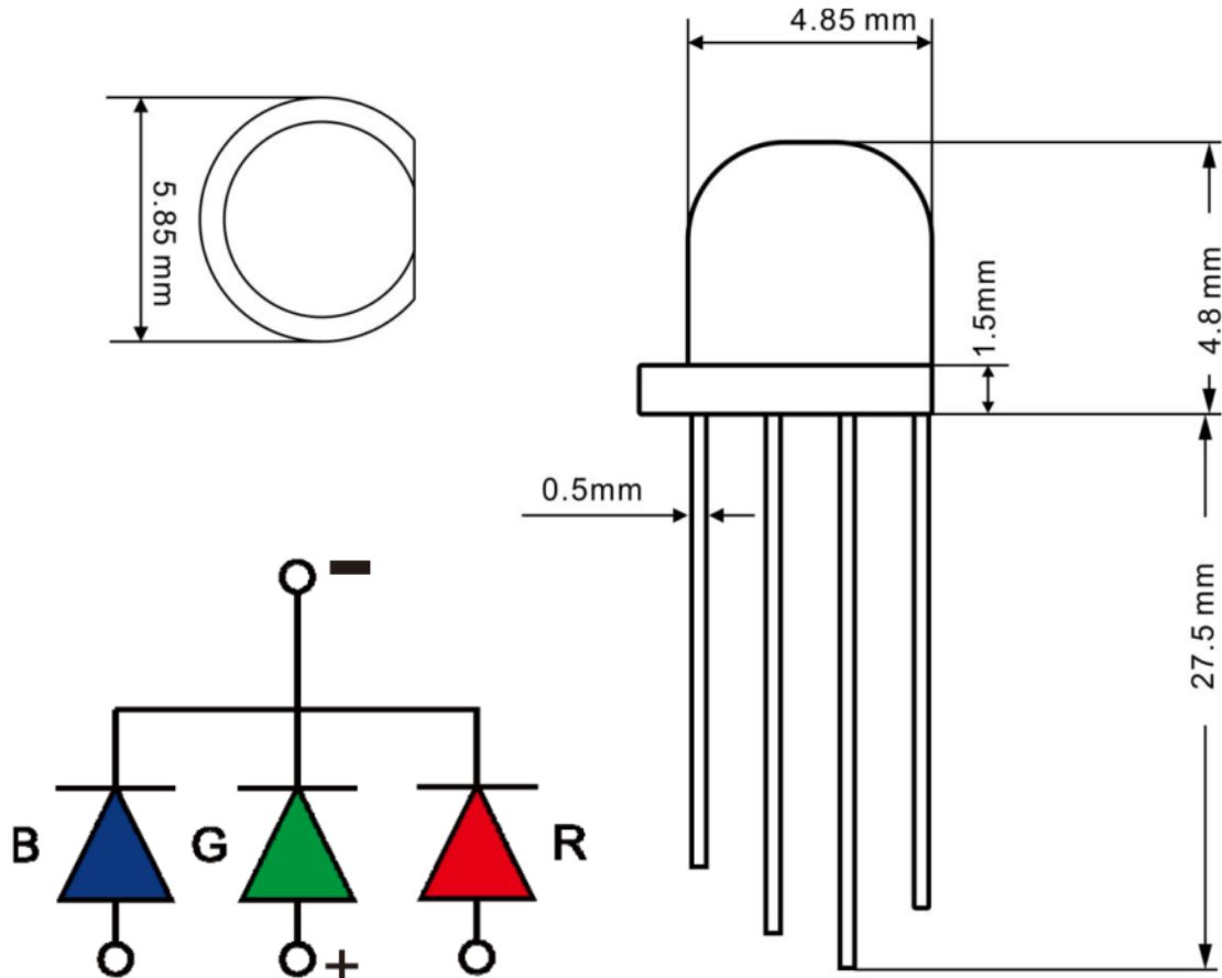
Emitter外型图:
