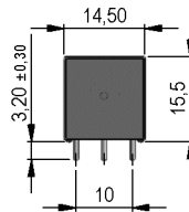
Layout Top view Draufsicht
