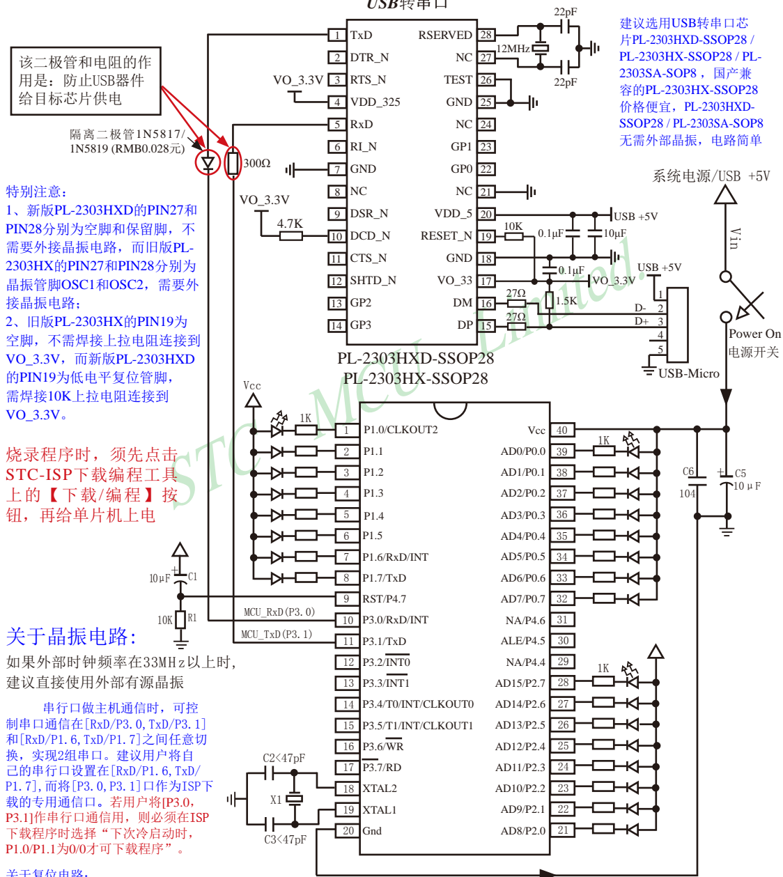
应用线路图
