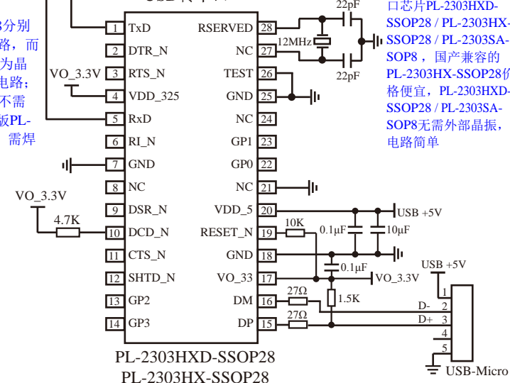
STC 单片机在线编程线路图 USB转串口
