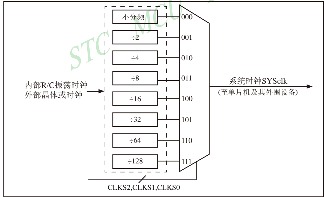
时钟结构
