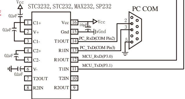
STC 单片机仿真应用线路图
