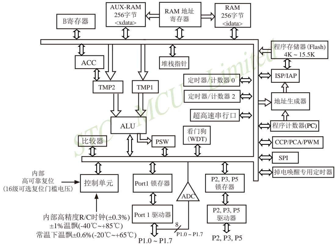
STC15W401AS系列内部结构框图
