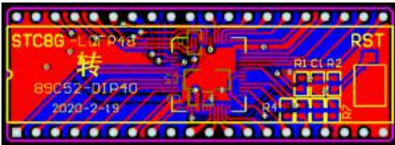
该转换板可进行 STC15H2K64S4 系列 LQFP48 转 STC89C52RC/STC89C58RD+ 系列仿真用。
