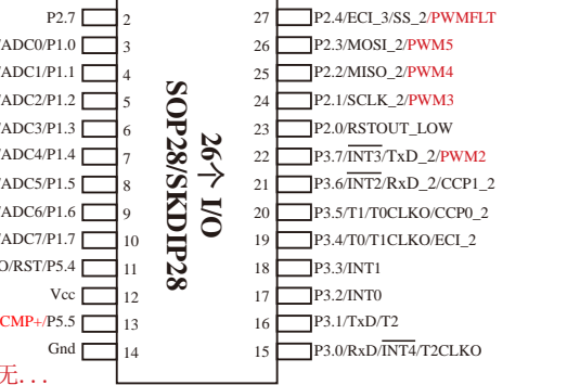
SOP28/SKDP28
