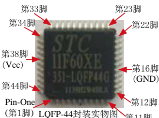
LQFP-44封装实物图
