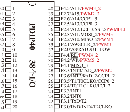
PDIP40 38 I/O
