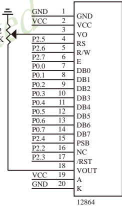
液晶模块 12864接口插座 R82、R83调整LCD背光亮度
