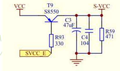
STC15系列单片机电路的电源控制部分参考电路图
