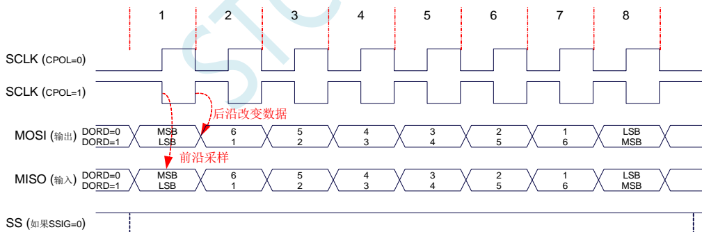
主机传输 (CPHA=0)
