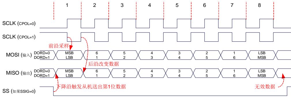
从机传输 (CPHA=0)
