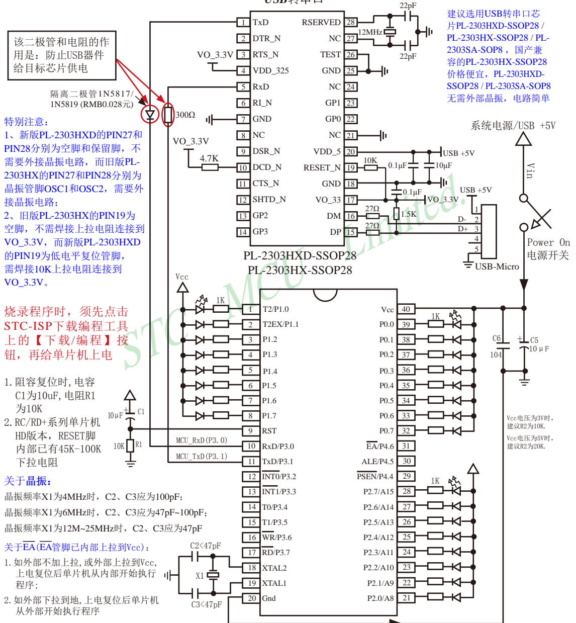
应用线路图
