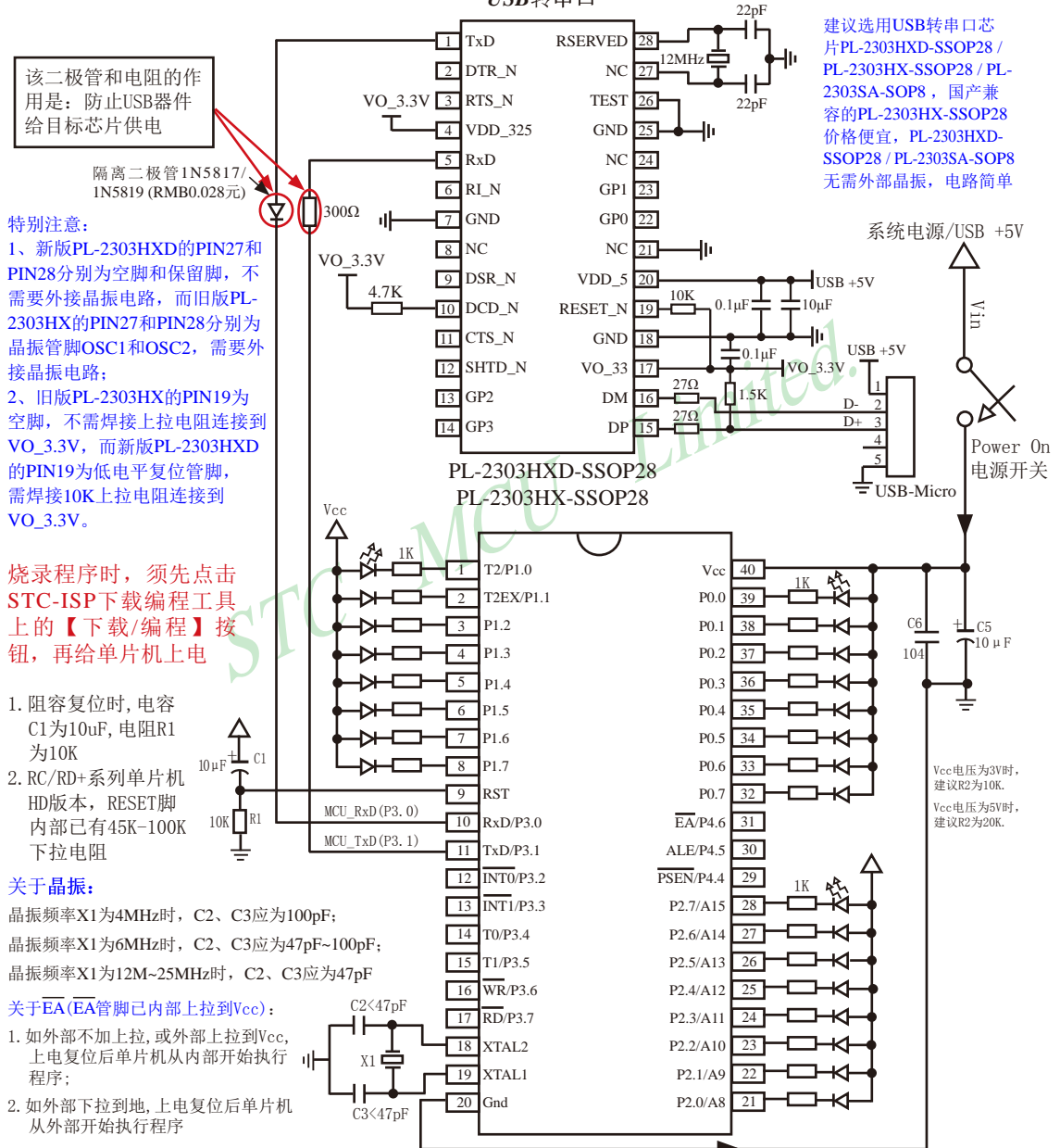
应用线路图
