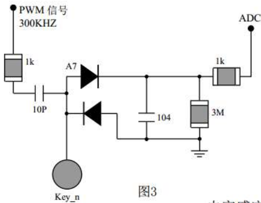
图3 电容感应按键取样电路
