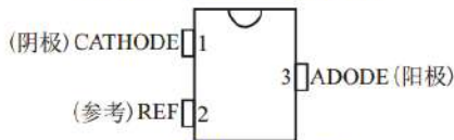
基准参考电压源TL431B
