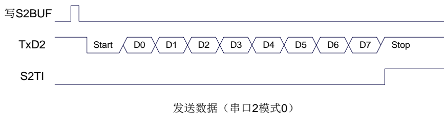
发送数据 (串口2模式0)
