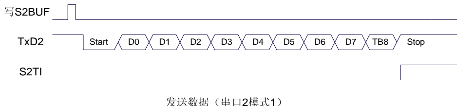
发送数据 (串口2模式1)
