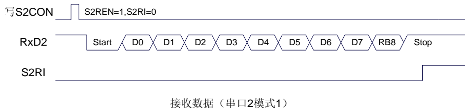
接收数据（串口2模式1）
