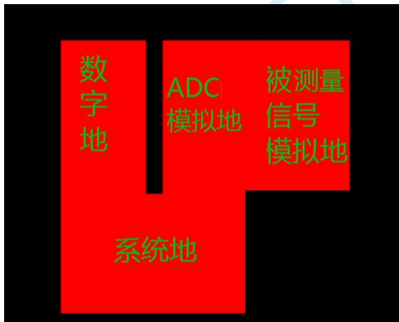
PCB 布线示意图
