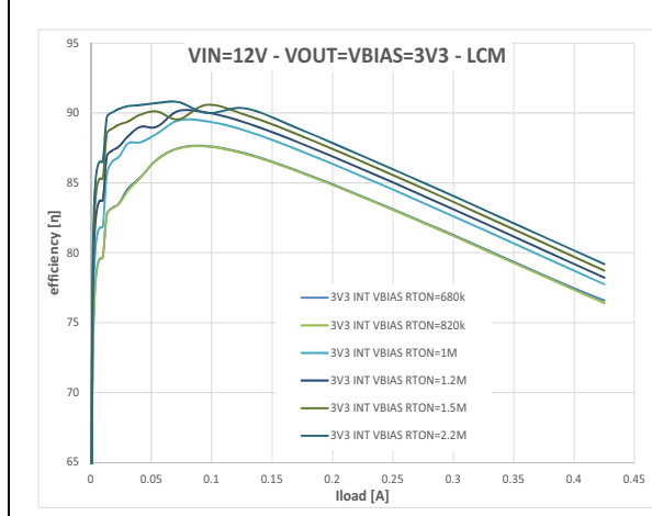
Figure 35. VIN 12 V - VOUT 3.3 V (linear scale)
