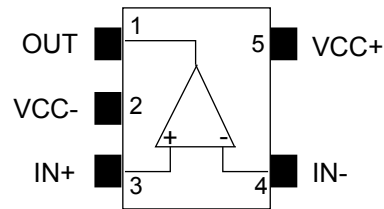
SOT23-5
