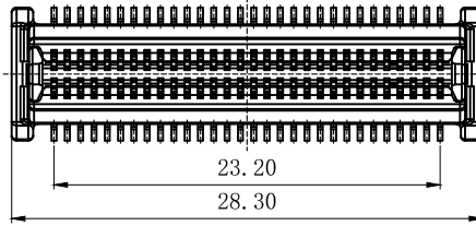
60PIN: BB41-60FT-1B-XHR
