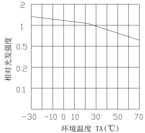
发光强度与环境温度
