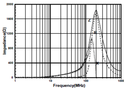
SBM1608G471GSP
