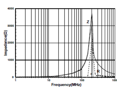
SBM1608G601GSP
