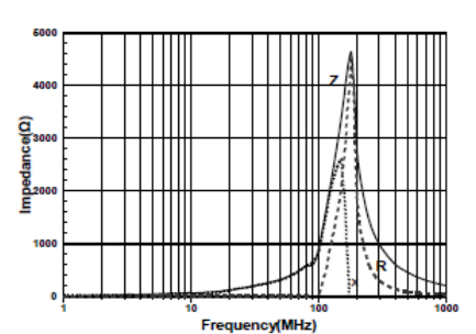
SBM1608G102ESP
