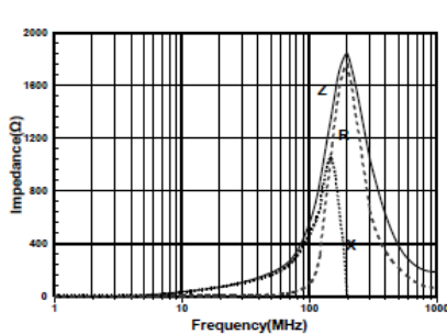
SBM1608G471GSP
