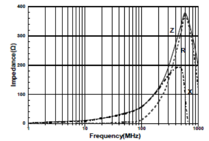
SBM2012G600JSP
