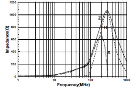
SBM2012G301HSP
