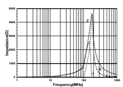
SBM1608G102ESP
