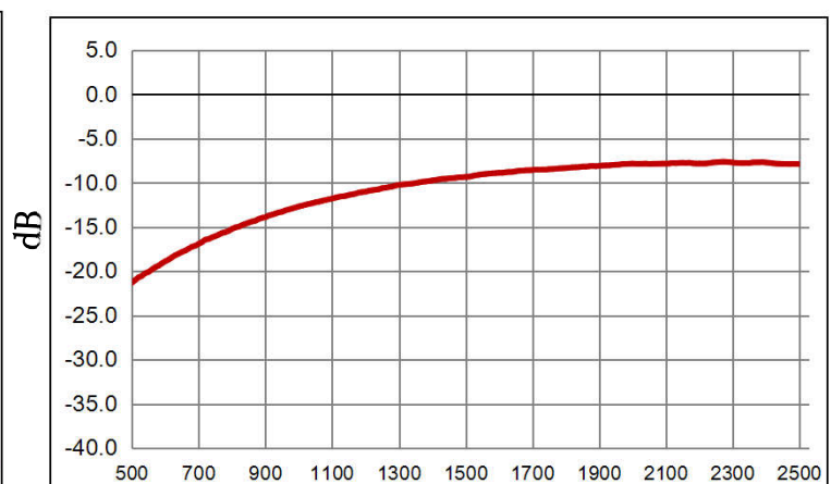
Sdd22
