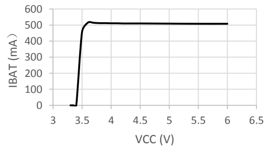
IBAT vs VCC
