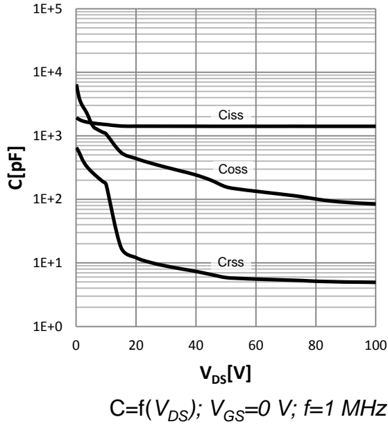
Typ. capacitances
