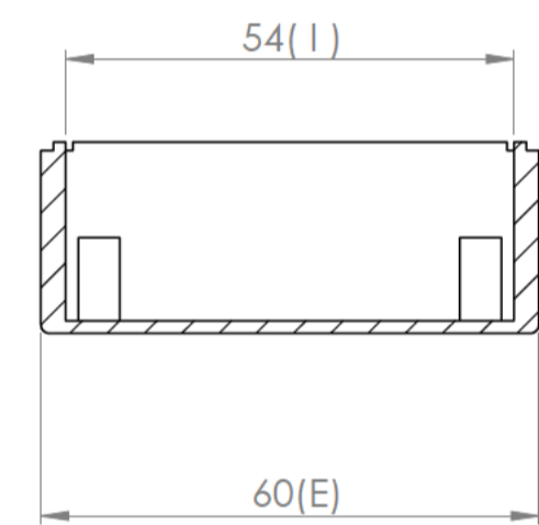
Seccio N-N / Section N-N
