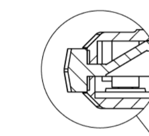
DETALLE/DETAIL R ESCALA 2 : 1
