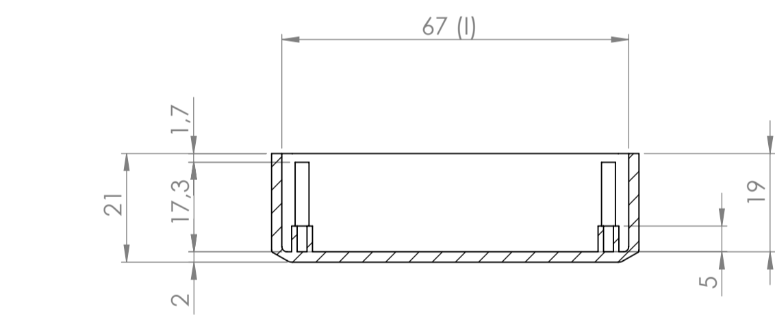
Sección D-D / Section D-D
