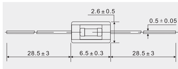
Dimensions(mm)尺寸
