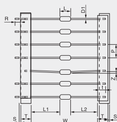
AXIAL TAPING 直線編帶
