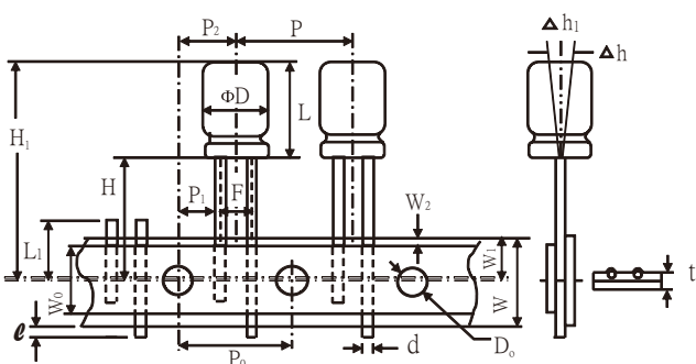
Fig.5( \phi 12-\phi 13 )
