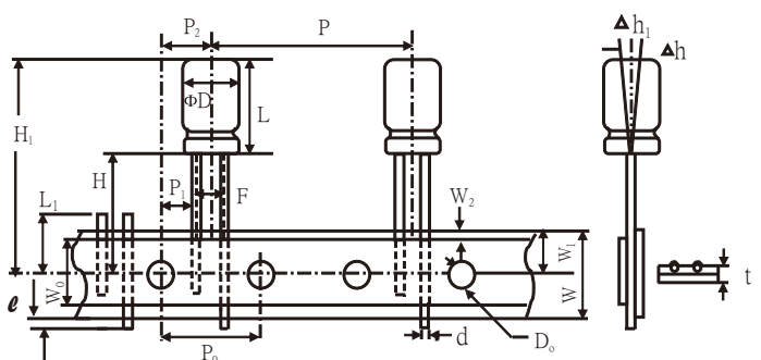
Fig.6( \phi 16 )
