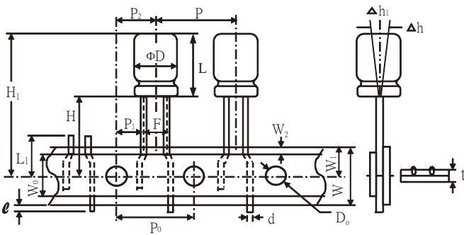
Fig.5(φ 12~φ 13)
