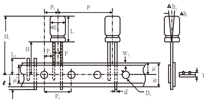
Fig.6(φ 16)
