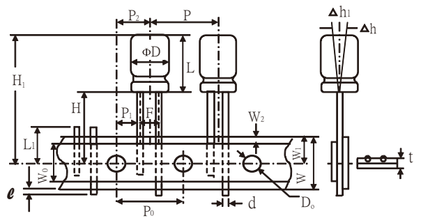
Fig.6(φ 16)
