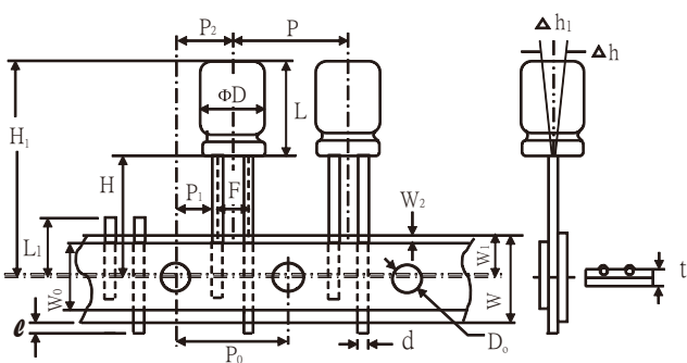
Fig.5(φ 12~φ 13)
