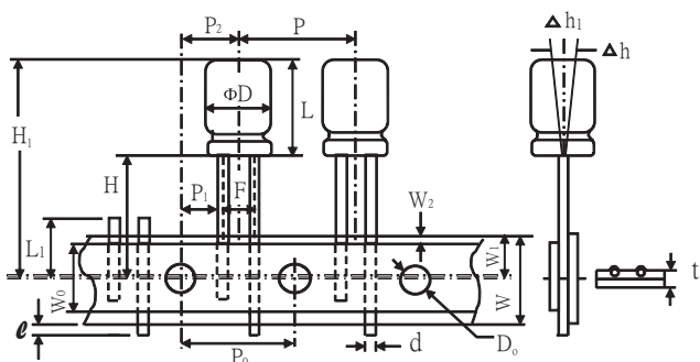
Fig.5(φ 12~φ 13)
