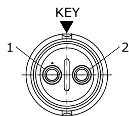
WIRING END W6382-2SG-P-5XX
