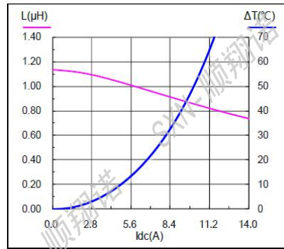
SMMS0530-2R2M
