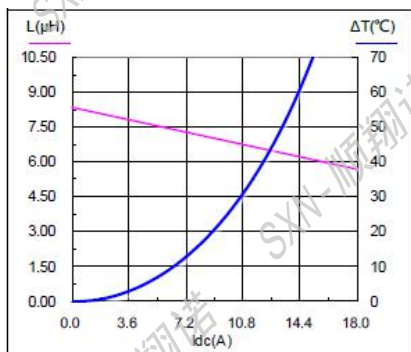
SMMS1360-8R2M
